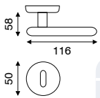
art. 1.8660 guarnitura rosetta e bocchetta ø 50 mm ad avvitare
