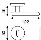
art. 1.5460 guarnitura rosetta e bocchetta ø 50 mm ad avvitare
