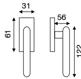
art. FI 2.4170 dk movimento in fibra con rosetta rettangolare 31x61 mm
