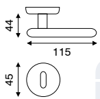
art. MA 2.476I guarnitura rosetta e bocchetta ø 45 mm a pressione
