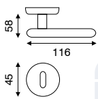
art. MA 2.286I guarnitura rosetta e bocchetta ø 45 mm a pressione
