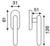
art. FI 2.2760 dk movimento in fibra
