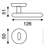
art. MA 2.2760 guarnitura rosetta e bocchetta ø 50 mm ad avvitare
