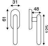
art. FI 2.1660 dk movimento in fibra
