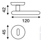
art. MA 2.6161 guarnitura rosetta e bocchetta ø 45 mm a pressione
