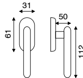
art. 4.7360 dk movimento in fibra
