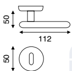
art. 1.7370 guarnitura rosetta e bocchetta bombata ø 50 mm ad avvitare
