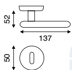
art. MA 2.3560 guarnitura rosetta e bocchetta ø 50 mm ad avvitare
