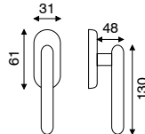
art. FI 2.246O dk movimento in fibra
