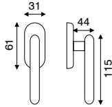
art. FI 2.476O dk movimento in fibra
