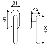
art. FI 2.456O BIC dk movimento in fibra
