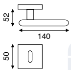
art. MA 2.5775 guarnitura rosetta e bocchetta quadra 50x50 mm
