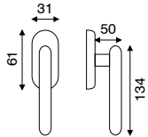
art. FI 2.756O dk movimento in fibra
