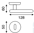
art. MA 2.1260 guarnitura rosetta e bocchetta ø 50 mm ad avvitare
