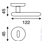
art. MA 2.456I BIC guarnitura rosetta e bocchetta ø 45 mm a pressione
