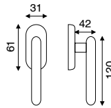
art. FI 2.6160 dk movimento in fibra
