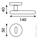
art. MA 2.5660 guarnitura rosetta e bocchetta ø 50 mm ad avvitare
