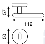
art. I.7270 guarnitura rosetta e bocchetta bombata ø 50 mm ad avvitare
