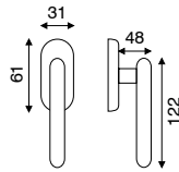
art. FI 2.3760 dk movimento in fibra
