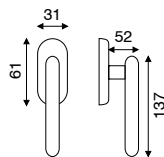
art. FI 2.3560 dk movimento in fibra
