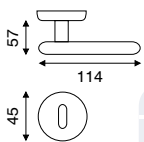
art. 1.9061 guarnitura rosetta e bocchetta ø 45 mm a pressione
