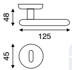
art. MA 2.1661 guarnitura rosetta e bocchetta ø 45 mm a pressione
