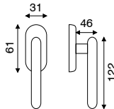
art. 4.5460 dk movimento in fibra
