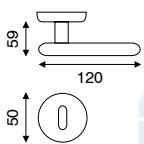
art. I.696O guarnitura rosetta e bocchetta ø 50 mm ad avvitare
