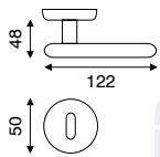
art. MA 2.3760 guarnitura rosetta e bocchetta ø 50 mm ad avvitare
