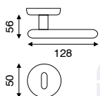
art. MA 2.4260 guarnitura rosetta e bocchetta ø 50 mm ad avvitare
