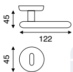
art. MA 2.456I guarnitura rosetta e bocchetta ø 45 mm a pressione
