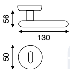
art. MA 2.3860 guarnitura rosetta e bocchetta ø 50 mm ad avvitare
