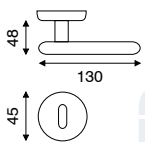
art. MA 2.246I guarnitura rosetta e bocchetta ø 45 mm a pressione
