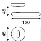
art. MA 2.7361 guarnitura rosetta e bocchetta ø 45 mm a pressione
