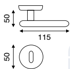
art. 1.2160 guarnitura rosetta e bocchetta ø 50 mm ad avvitare
