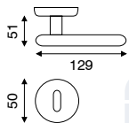
art. MA 2.3060 guarnitura rosetta e bocchetta ø 50 mm ad avvitare
