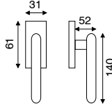
art. FI 2.5770 dk movimento in fibra con rosetta rettangolare 31x61 mm
