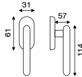
art. 4.9060 dk movimento in fibra
