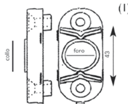
Art. 9.0062 Movimento DK speciale con viti (movimento (1) + rotore (2) che è quello che fa scattare il movimento)
