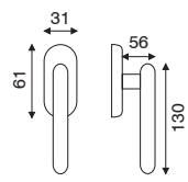
art. FI 2.3860 dk movimento in fibra
