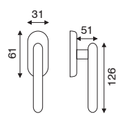
art. FI 2.2760 dk movimento in fibra
