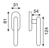
art. FI 2.5060 dk movimento in fibra
