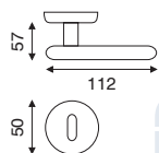
art. I.7270 guarnitura rosetta e bocchetta bombata ø 50 mm ad avvitare
