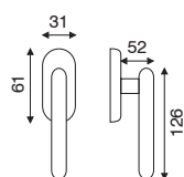
art. FI 2.3260 dk movimento in fibra
