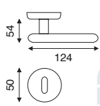
art. MA 2.5070 guarnitura rosetta e bocchetta bombata ø 50 mm ad avvitare
