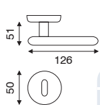
art. MA 2.2760 guarnitura rosetta e bocchetta ø 50 mm ad avvitare
