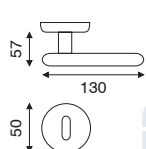
art. MA 2.1560 guarnitura rosetta e bocchetta ø 50 mm ad avvitare
