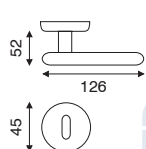
art. MA 2.3261 guarnitura rosetta e bocchetta ø 45 mm a pressione
