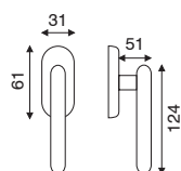
art. FI 2.2260 dk movimento in fibra
