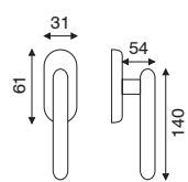
art. FI 2.4960 dk movimento in fibra
