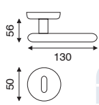
art. MA 2.3860 guarnitura rosetta e bocchetta ø 50 mm ad avvitare
