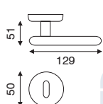
art. MA 2.3060 guarnitura rosetta e bocchetta ø 50 mm ad avvitare
