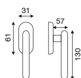
art. FI 2.1760 dk movimento in fibra
