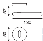
art. MA 2.1772 guarnitura rosetta e bocchetta bombata ø 50 mm ad avvitare
