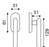
art. FI 2.3060 dk movimento in fibra
