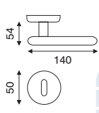
art. MA 2.4970 guarnitura rosetta e bocchetta bombata ø 50 mm ad avvitare
