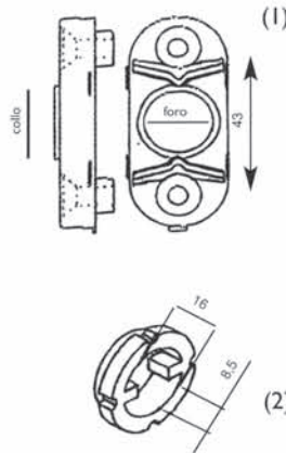
Art. 9.0062 Movimento DK speciale con viti (movimento (1) + rotore (2) che è quello che fa scattare il movimento)
