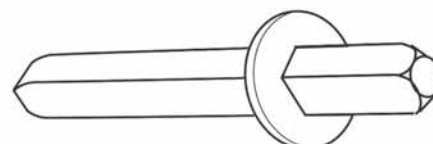
Art. 9.0045 Ferro \square 7 con rondella per martelline conf. pz. 50
